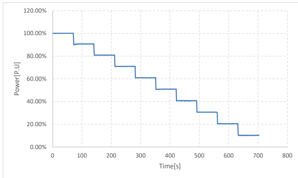
Gráfico limitação da potência activa em coincidência com comando remoto Graph active power limitation in adjusted with remote contro
